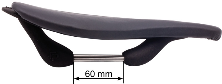
Abbildung 3: Abmessungen des Sattelgestells
